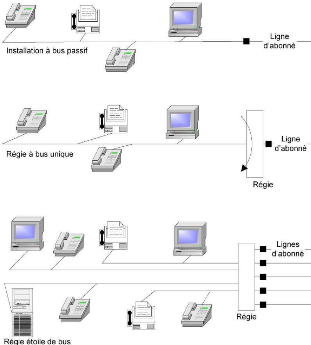
La régie à étoile de bus permet de raccorder en étoile jusqu'à 64 terminaux
