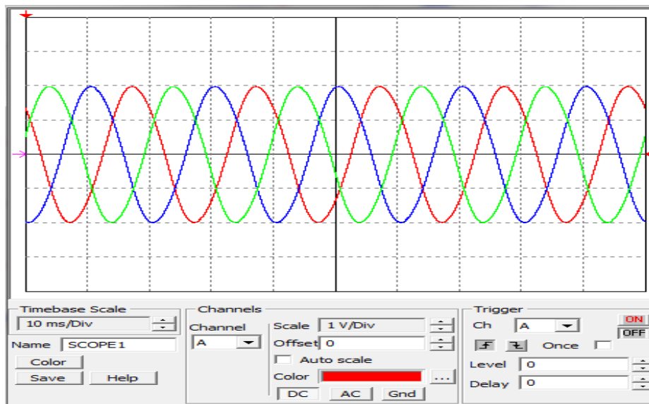
Figure 26 : La forme du courant dans la charge triphasée après filtrage
