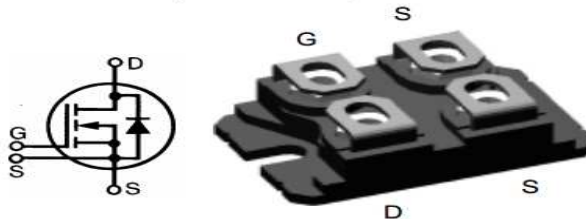
Figure 52 : Caractéristiques du Mosfet IXFE 36N100
