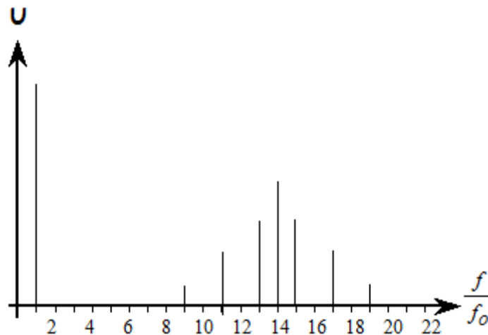
Figure 12 : Spectre unilatérale du signal de sortie de l'onduleur
