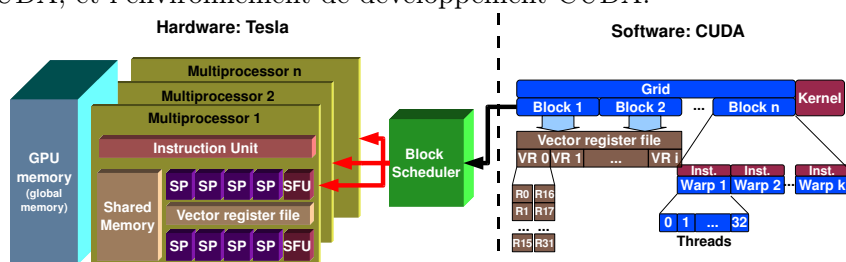
FIGURE 1.2 – Description de l'architecture TESLA.
